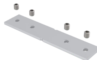
LACZ-AST-PZ-SN-01W Łącznik płaski prosty + 4 wkrety do Japet, Japet XL, Fobos, Fobos XL Flat connector + 4 screws for Japet, Japet XL, Fobos, Fobos XL Gerader Flachverbinder + 4 Schrauben für Japet, Japet XL, Fobos, Fobos XL 5908293402882
